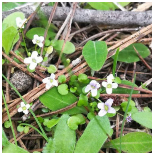
Fotografia 5.6 – Jonopsidium acaule observado na área em estudo
