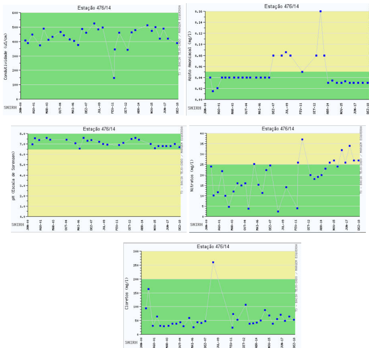
Figura 5.26 – Evolução da Qualidade da água na estação de monitorização 476/14
