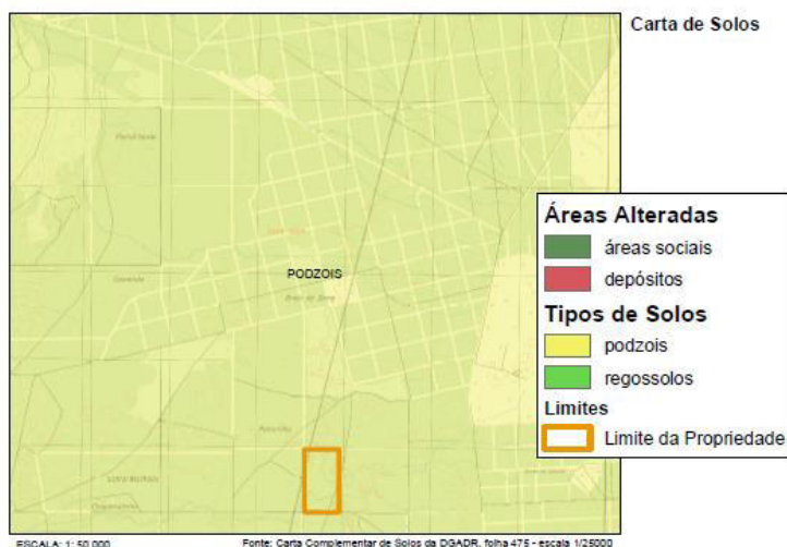
Figura 5.35 – Classificação dos Solos na área de inserção do projeto
