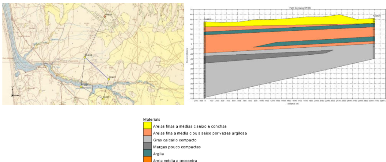
Figura 5.13 – Perfil geológico NW-SE entre os furos RAQ018 e RAQ020 constantes da base de dados da Rios&Aqüíferos e respetiva localização na Carta Geológica de Portugal à escala 1/50 000 Folha 39-C Alcácer do Sal.
