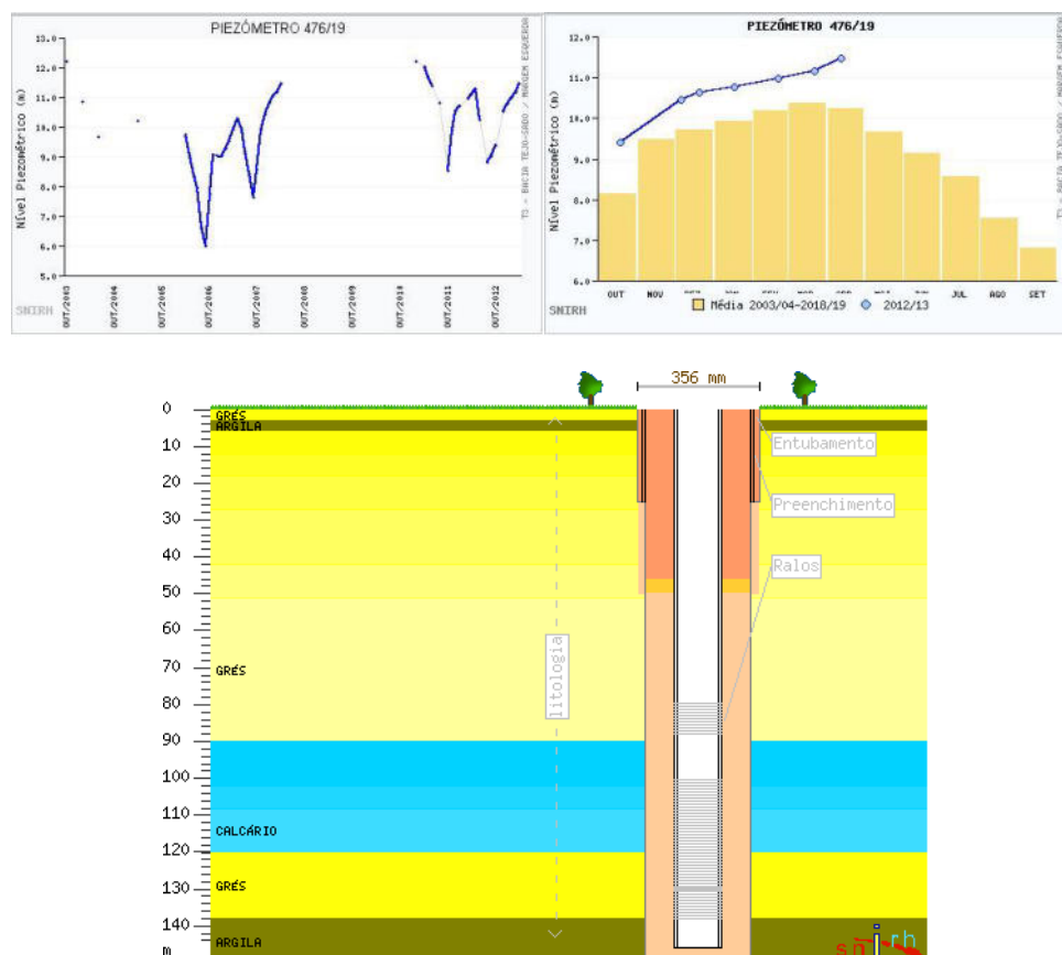
Figura 5.21 – Estação de monitorização 476/19 – Evolução do nível piezométrico
