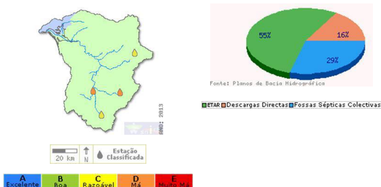
Figura 5.19 – Classificação da qualidade da água para fins múltiplos na bacia do rio Sado (2013)
