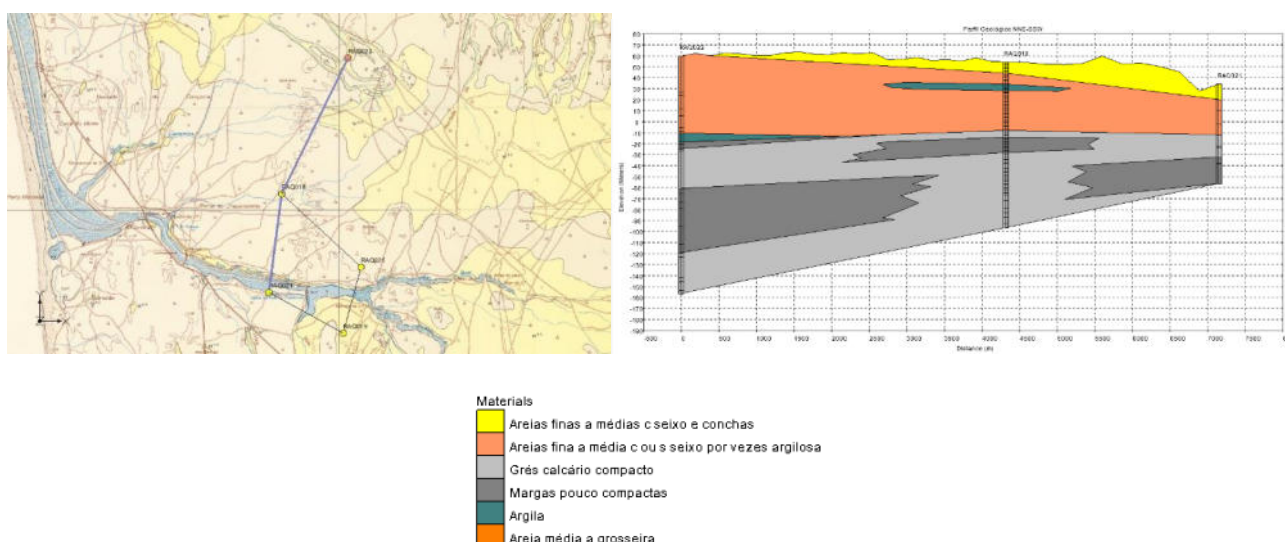
Figura 5.12 – Perfil geológico NNE-SSW entre os furos RAQ022, RAQ018 e RAQ021 constantes da base de dados da Rios&Aqüíferos e respetiva localização na Carta Geológica de Portugal à escala 1/50 000 Folha 39-C Alcácer do Sal.
