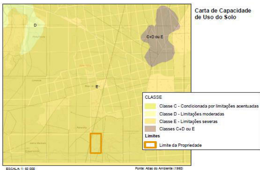
Figura 5.36 – Capacidade de Uso dos Solos na área de inserção do projeto
